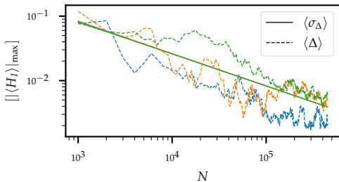
Mean Actual vs. Allowed deviation.
