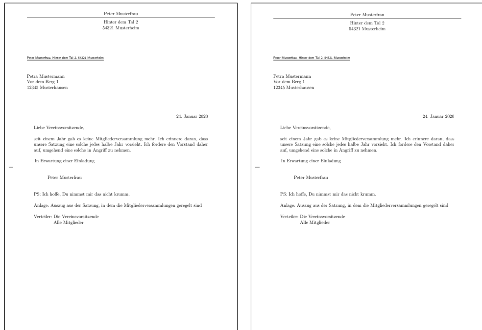
Abbildung 4.13.: Ergebnis eines kleinen Briefes mit Absender, Trennlinie, Anschrift, Anrede, Text, Grußfloskel, Signatur, Postskriptum, Anlagen, Verteiler und Lochermarke (das Datum entstammt den Voreinstellungen für DIN-Briefe); links der einfache Briefkopf mit fromalign=false , rechts der erweiterte Briefkopf mit fromalign=center
