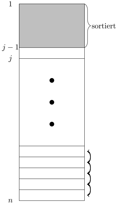
Bubblesort
