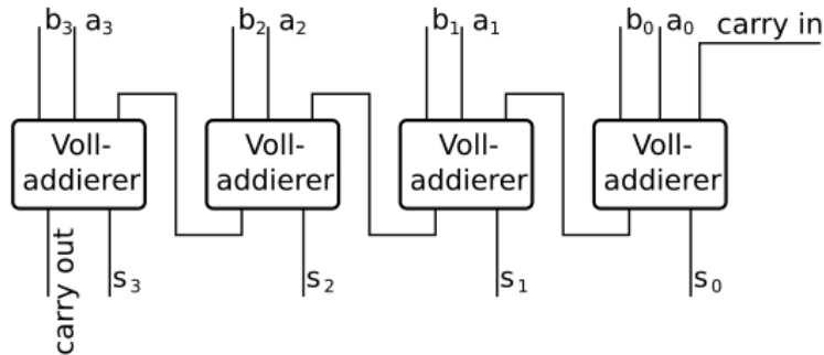
Abbildung V.3: Carry-Ripple-Adder
